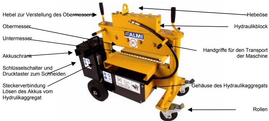
Abbildung 4.2-1: Aufbau der Maschine
