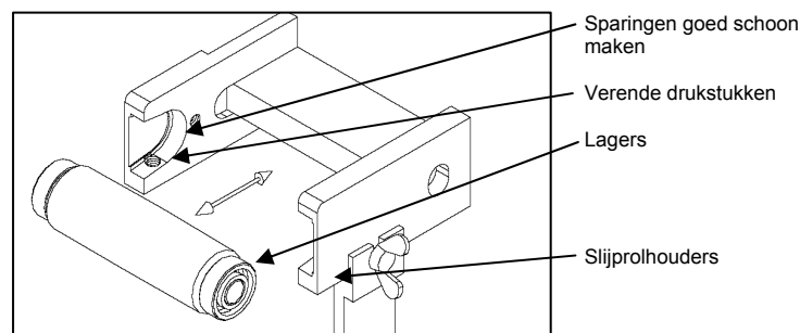
Figuur 4.6-4: Verwisselen slijprol
