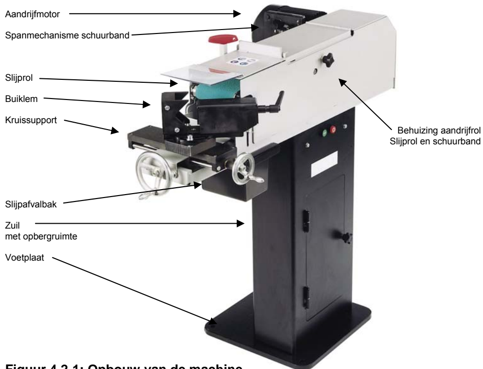
Figuur 4.2-1: Opbouw van de machine
