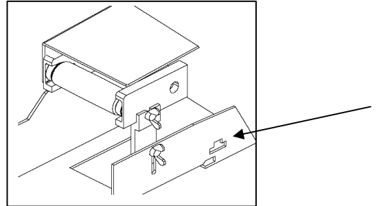
Figuur 4.6-2: Steun slijprolhouder
